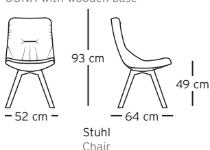
JONA mit Holzuntergestell JONA with wooden base
