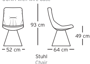
JONA mit Drahtuntergestell JONA with wire base
